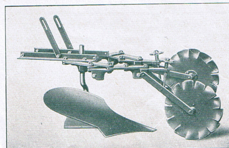
Fig. 4. — Montage du soc de charrue. Le soc de charrue se place toujours à l'avant, la roue motrice marche derrière le soc, dans le fond de la raie.
