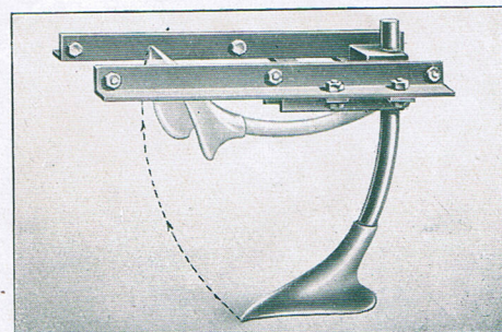
Fig. 8. — Châssis spécial sous-soleur se montant à l'arrière. Prix : 240. »
