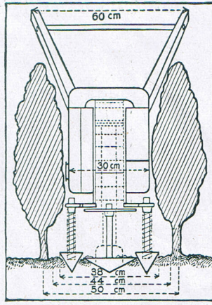
Fig. 9. — Façonnage et binage de plants hauts en ligne à 0 m. 50.
