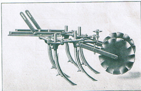
Fig. 1. — Montage des outils cultivateurs à l'avant. Dans les cultures en lignes employez de préférence les outils montés à l'avant.
