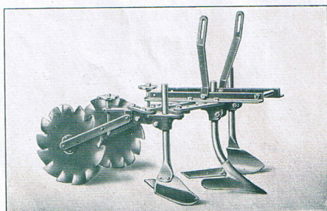
Fig. 7. — Montage à l'arrière de deux rasettes et d'une patte d'oie. Deux paires de rasettes peuvent être montées.
