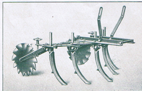
Fig. 2. — Montage des outils cultivateurs sur le châssis placé à l'arrière. Pour travailler des terres en jachère, les outils peuvent être montés à l'arrière, comme l'indique le cliché ci-dessus.
