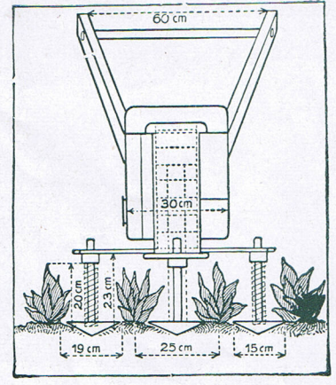
Fig. 10. — Les outils peuvent se placer à des écartements différents.
