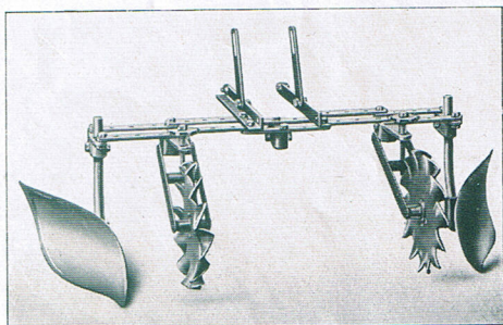
Fig. 5. — Montage des versoirs à l'avant. Ces versoirs peuvent être inversés pour débutter. Sur le cliché ci-dessus, ils buttent.
