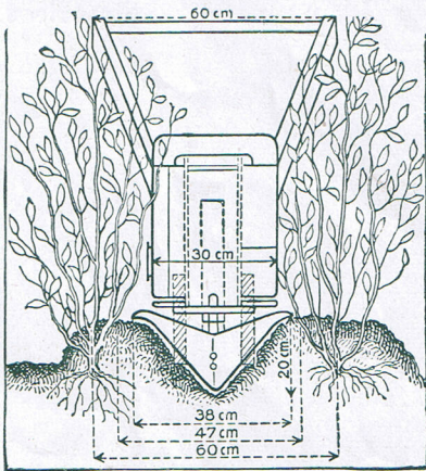
Fig. 8. — Buttage de plantes hautes : maïs, pommes de terre, arbustes, etc.
