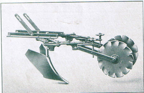
Fig. 3. — Montage du buttoir. Le buttoir peut être utilisé également pour billonner ou recouvrir les plants. Il se monte sur le châssis placé à l'avant.
